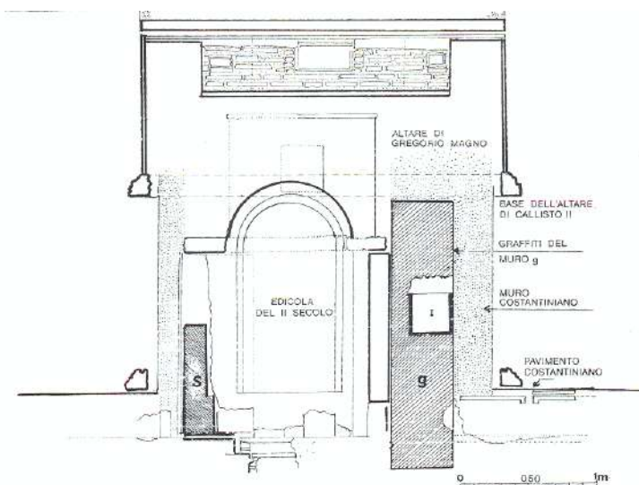
IV. Spaccato dei monumenti esistenti sotto l'altare della Confessione.
